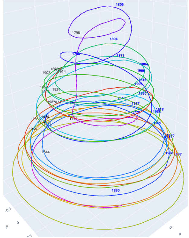
FIG. 4: Attracteur empirique, reconstruit à partir des séries temporelles du nombres de taches solaires par mois ( N = 2735 paires (x_i, y_i) observées). Les années des maxima solaires sont indiquées en bleu, les années de minima en noir. Une version dynamique, navigable, de cette structure est disponible en ligne à cette adresse : https://team.inria.fr/comcausa/continuous-causal-states/ .
